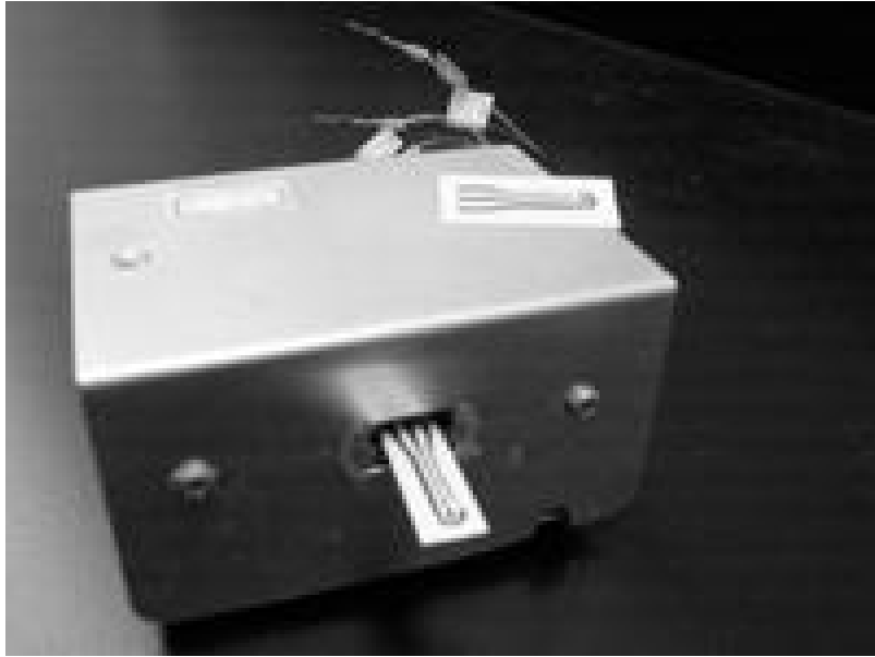
林孟山自製的恆電位儀，輕巧的體積，方便隨身攜帶做各種檢測。（記者邱湘媛攝）
