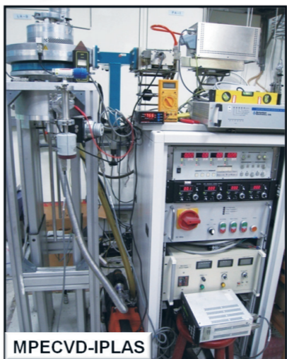
MPECVD-IPLAS
